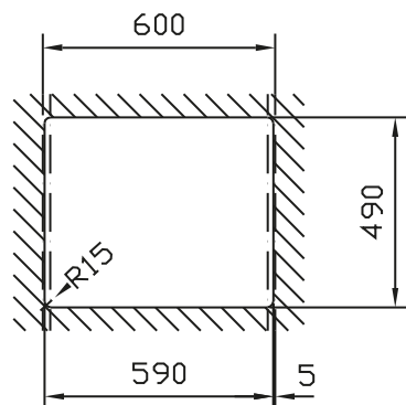
Ausschnitt übergreifend 1:20
