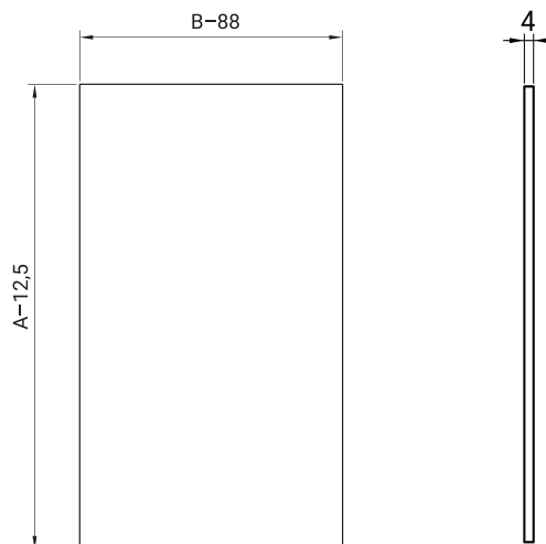
Габариты вставки
